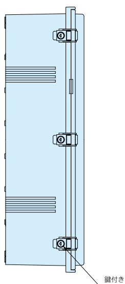
A矢視図 鍵付きラッチBCAK・BCPKシリーズ
