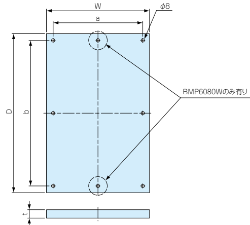
BMP5060W～6080W外観寸法図
