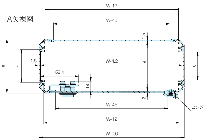
W方向図
