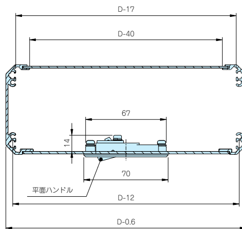
D方向図
