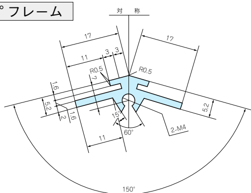
165° フレーム
