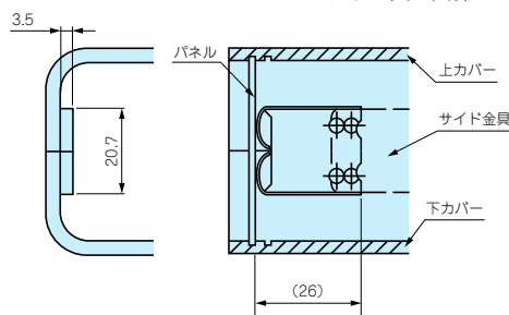
取付図
