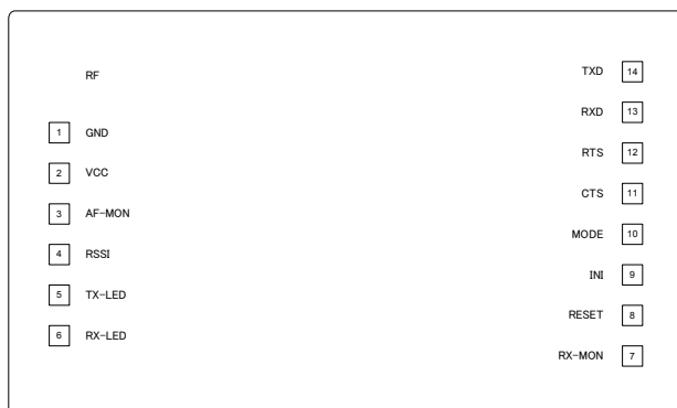
MU-1N 端子名、端子番号 (Top View)
