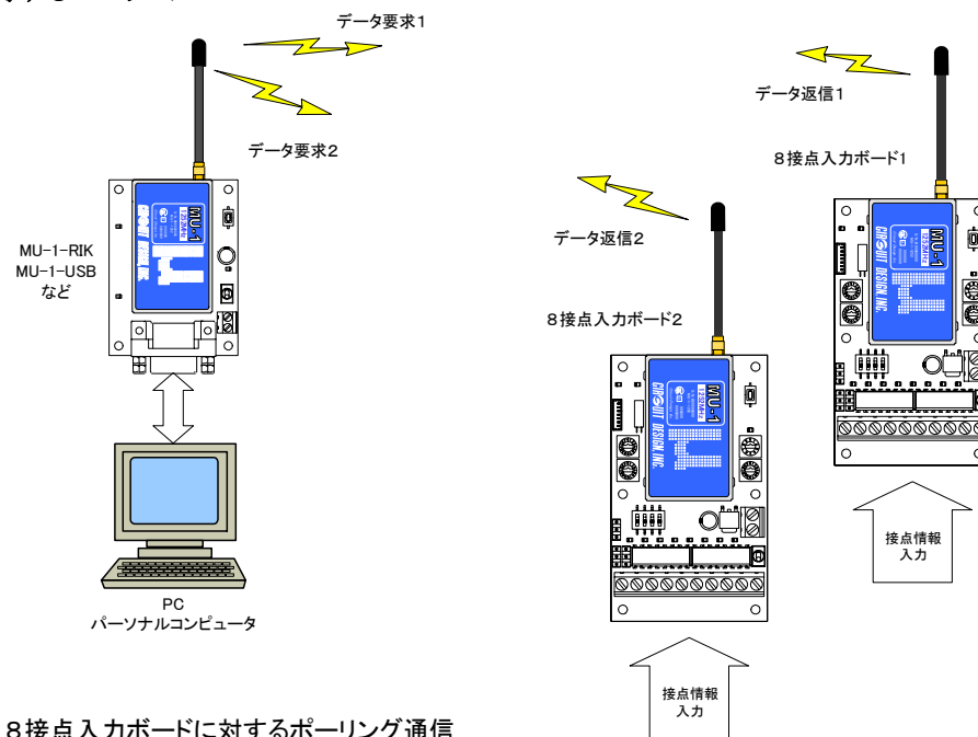
8接点入力ボードに対するポーリング通信
