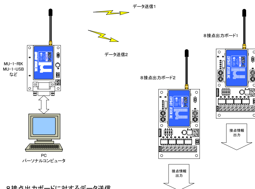
8接点出力ボードに対するデータ送信
