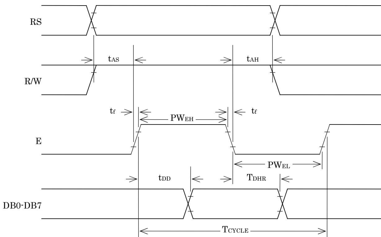
Figure 2. Motorola M68-Type パラレル 読み込みタイミング
