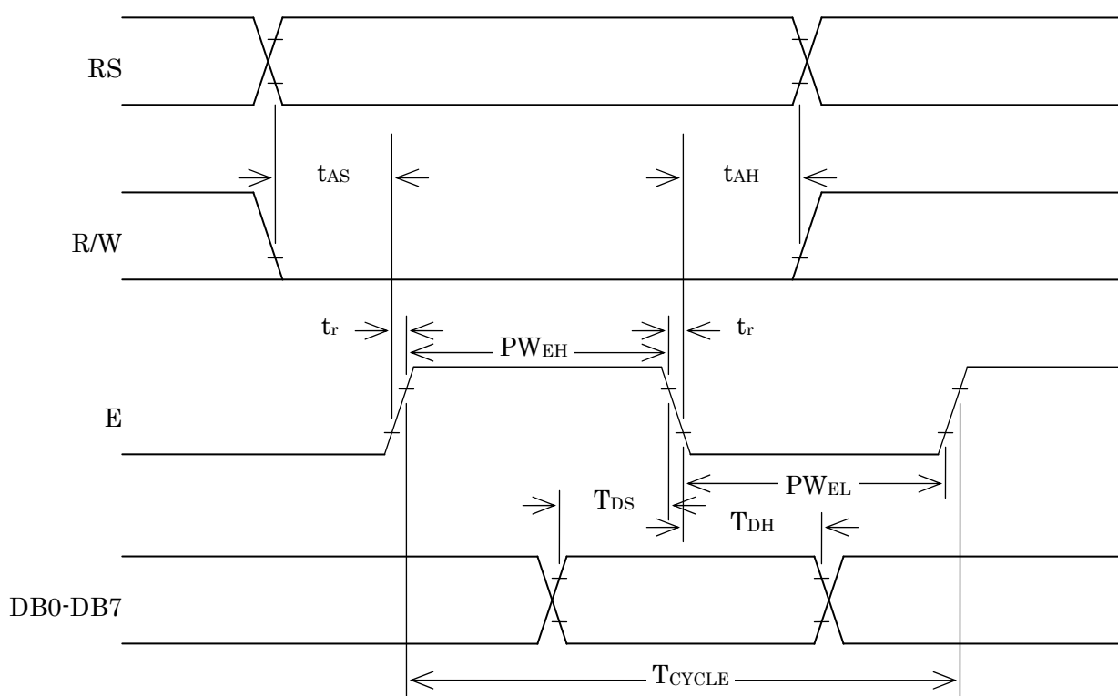
Figure 1. Motorola M68-Type パラレル 書き込みタイミング
