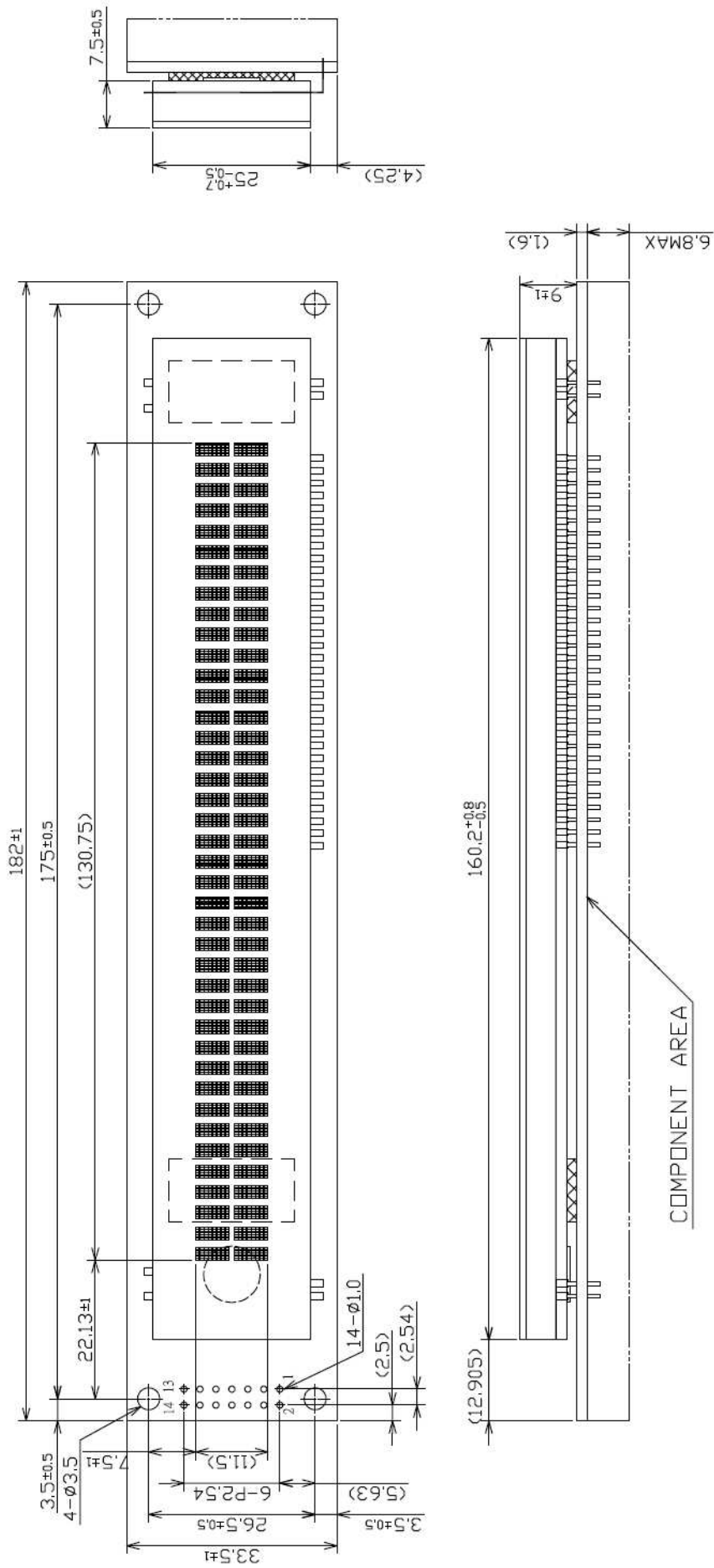
M402SD62AA 外形图
