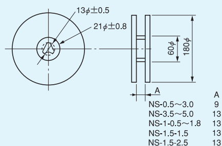
リール寸法図
