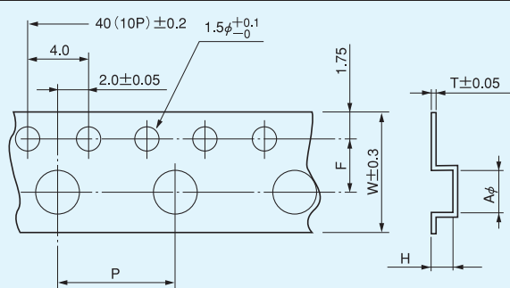
テープ寸法図
