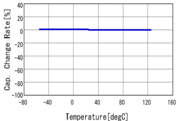
温度特性
