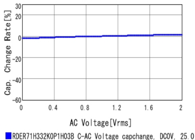
AC電圧特性
