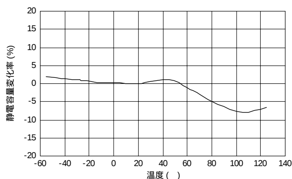
静電容量 - 温度特性 R1特性の例
