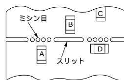
[基板ブレイク近辺でのコンデンサ配置]
