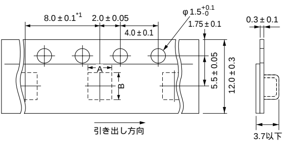
12mm幅8mm/4mmピッチテープ
