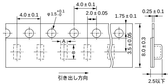
8mm幅4mmピッチテープ
