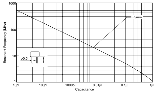
静電容量-共振周波数
