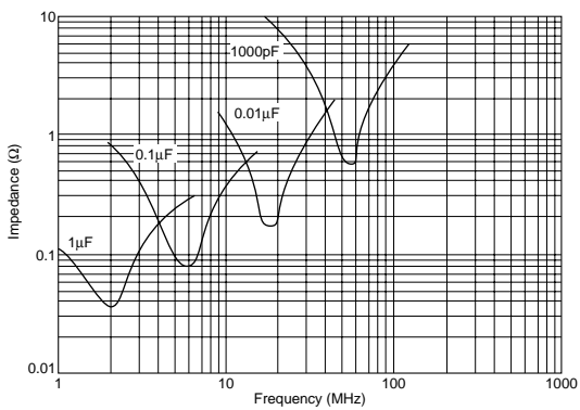
インピーダンス-周波数特性
