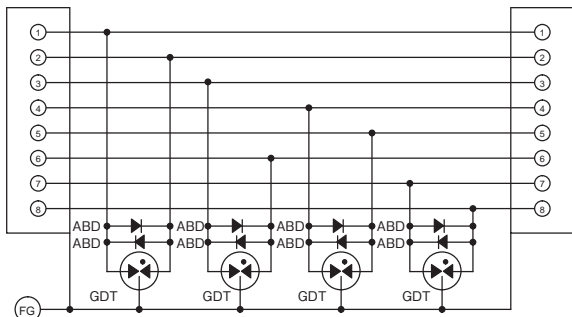
モジュラージャック (RJ45)
