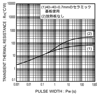
Fig.11 過度熱抵抗
