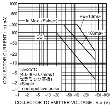
Fig.10 安全動作領域
