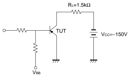
Fig.12 スイッチング特性測定回路
