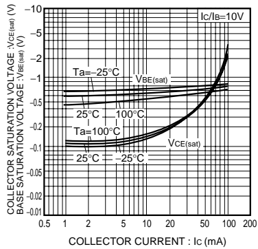
Fig.7 コレクタ・エミッタ間飽和電圧-ベース・エミッタ間飽和電圧-コレクタ電流特性
