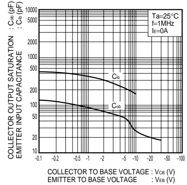
Fig.6 コレクタ出力容量-コレクタ・ベース間電流特性 エミッタ入力容量-エミッタ・ベース間電流特性
