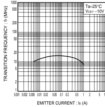
Fig.5 利得帯域幅積-エミッタ電流特性
