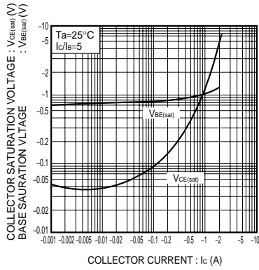
Fig.4 コレクタ・エミッタ間飽和電圧-コレクタ電流特性 ベース・エミッタ間飽和電圧-コレクタ電流特性
