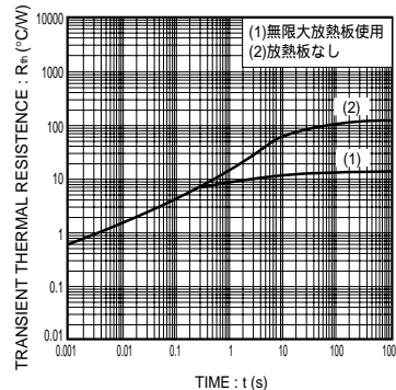
Fig.8 過度熱抵抗
