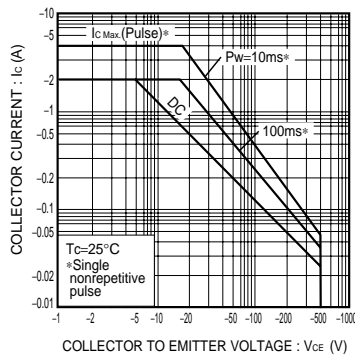
Fig.7 安全動作領域
