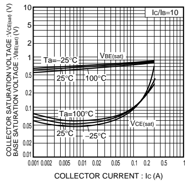
Fig.6 コレクタ・エミッタ間飽和電圧-コレクタ電流特性 ベース・エミッタ間飽和電圧-コレクタ電流特性
