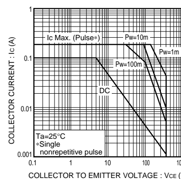
Fig.9 安全動作領域
