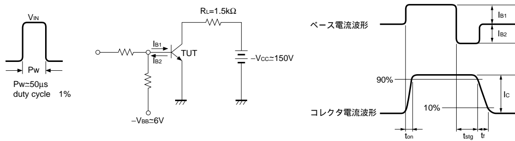
Fig.10 スイッチング時間測定回路図
