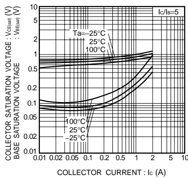
Fig.6 コレクタ・エミッタ間飽和電圧 - コレクタ電流特性 ベース・エミッタ間飽和電圧 - コレクタ電流特性
