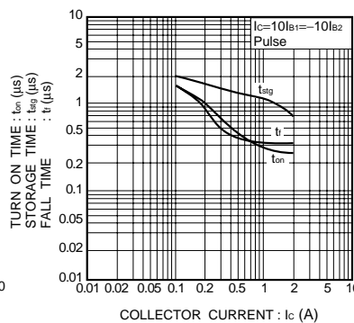
Fig.9 スイッチング時間 - コレクタ電流特性
