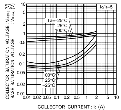
Fig.6 コレクタ・エミッタ間飽和電圧 - コレクタ電流特性 ベース・エミッタ間飽和電圧 - コレクタ電流特性
