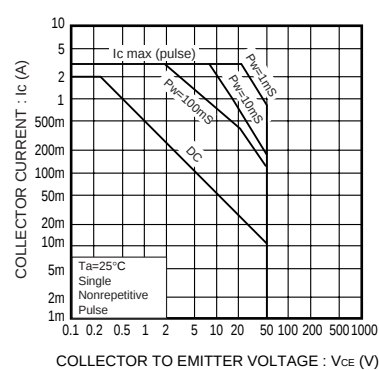
Fig.9 安全動作領域 (A. S. O) 2SD2212 (MPT)
