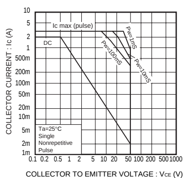
Fig.10 安全動作領域 (A. S. O) 2SD2143 (CPT)
