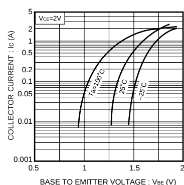
Fig.3 エミッタ接地伝達静特性
