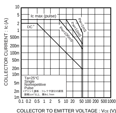
Fig.11 安全動作領域 (A. S. O) 2SD1866 (ATV)
