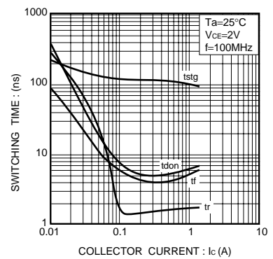
Fig.6 スイッチング時間
