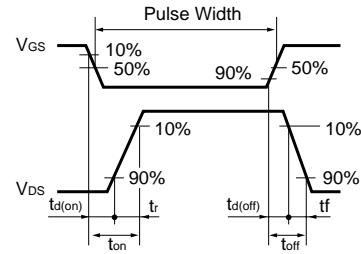
Fig.11 スイッチング波形
