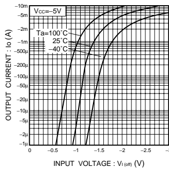
Fig.2 出力電流 - 入力電圧 (OFF特性)
