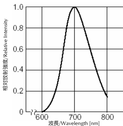
スペクトル分布特性 Relative Intensity vs. Wavelength 条件/Condition : T_a = 25^\circ\text{C} , I_f = 10\text{mA}
