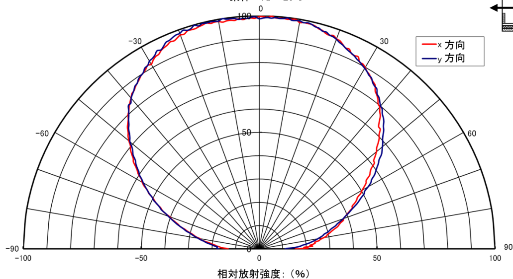
指向特性図
