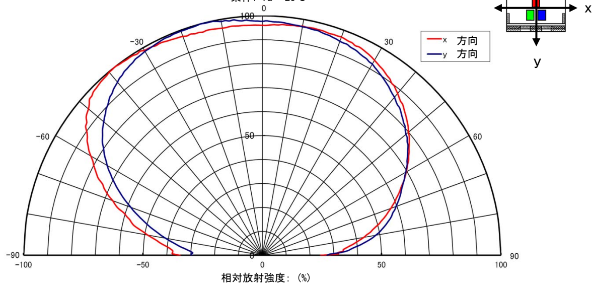
指向特性図
