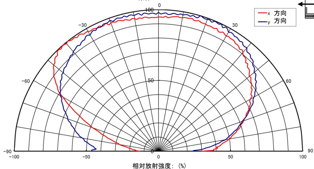
指向特性図
