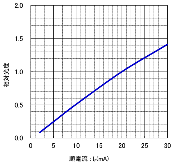
順電流－相対光度 特性
