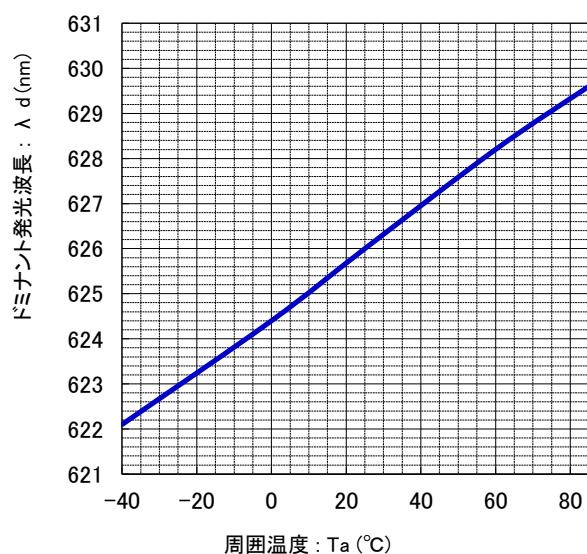
周囲温度－ドミナント波長 特性
