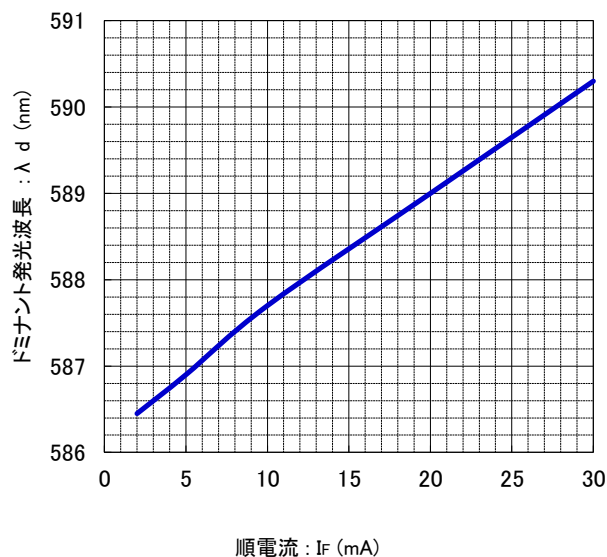
順電流－ドミナント波長 特性
