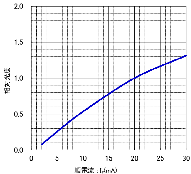
順電流－相対光度 特性
