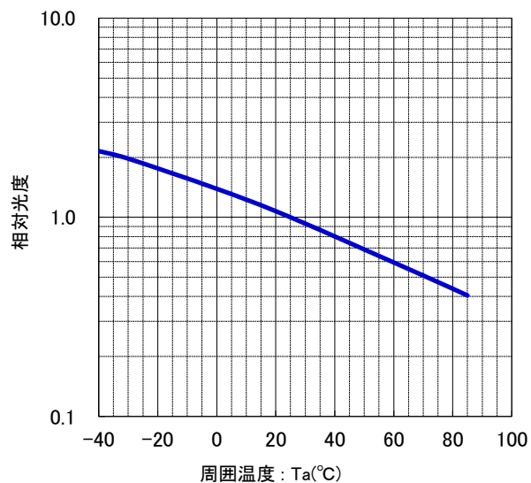
周囲温度－相対光度 特性
