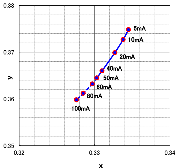
順電流 vs. 色度 特性
