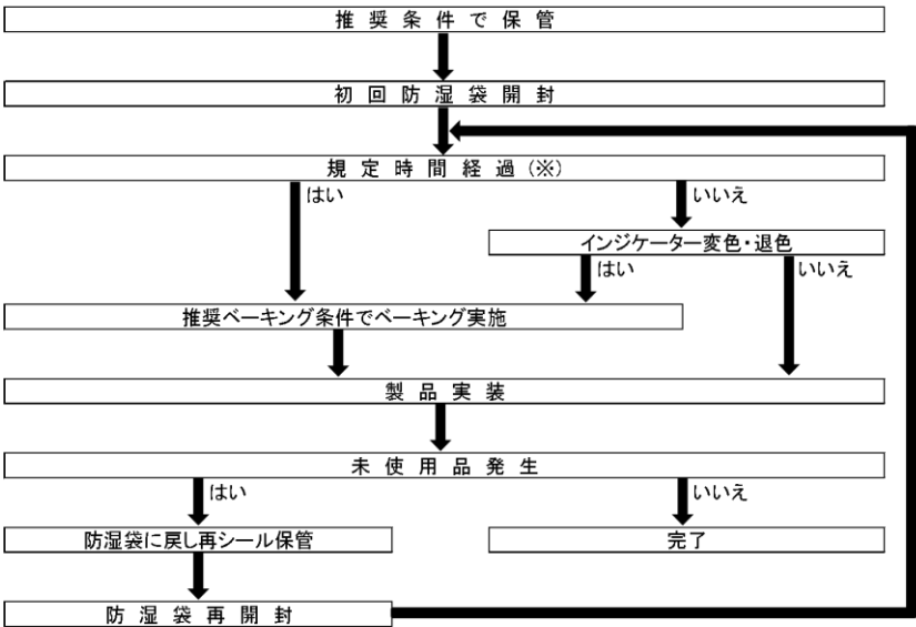
防湿袋開封から製品実装までのフロー概略
