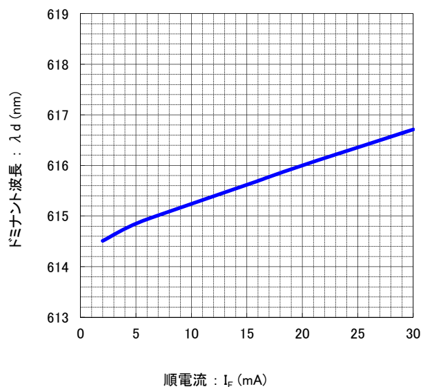
順電流ードミナント波長 特性
