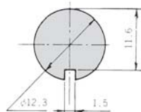
ロッキングリングを使用しない場合 Without Locking Ring
