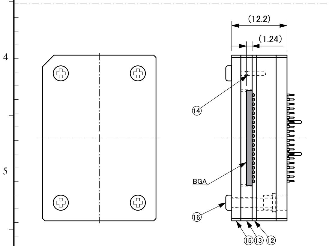
BGA搭載時(2/1)
