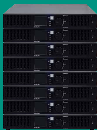
TOWER 40kW 高さ: 528 mm (12U) 重量: 144kg
