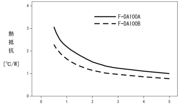
F-DA100A、F-DA100B 熱抵抗 (強制空冷)
