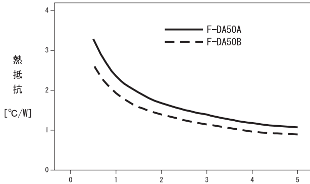
F-DA50A、F-DA50B 熱抵抗 (強制空冷)
