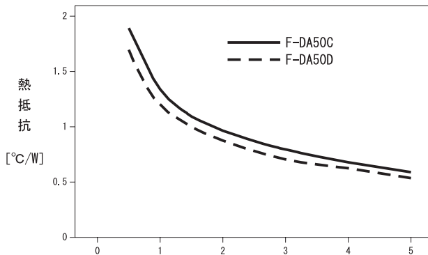
図2 F-DA50C、F-DA50D ヒートシンク熱抵抗
