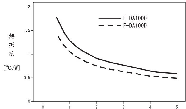
図4 F-DA100C、F-DA100D ヒートシンク熱抵抗
