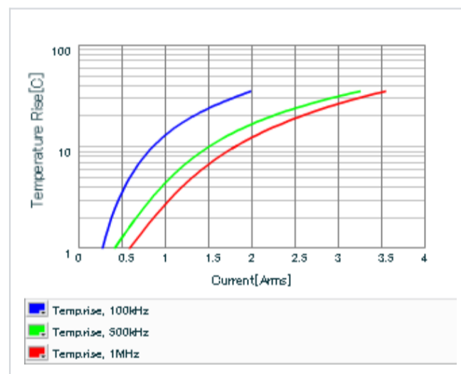
■ リップル発熱特性
