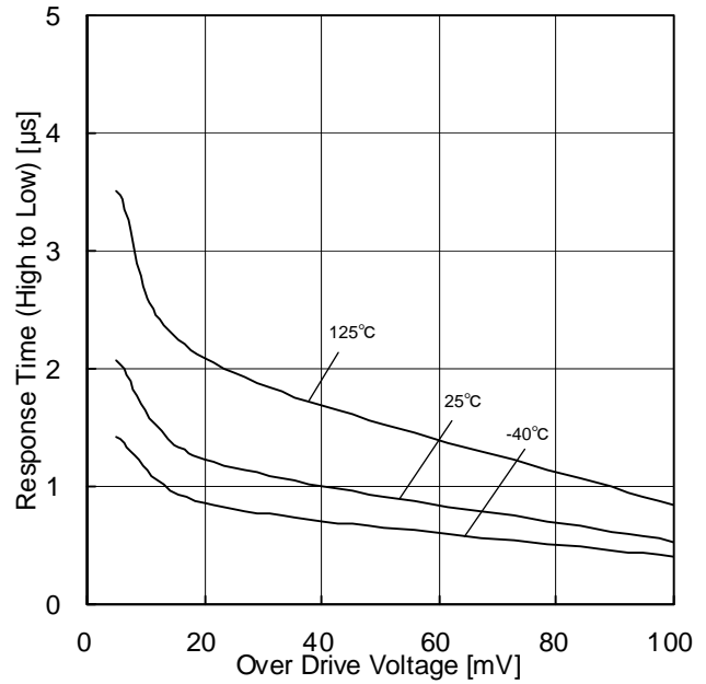
Figure 46. H→L 応答時間-オーバードライブ電圧特性 (VCC=5V, V RL =5V, R L =5.1kΩ)
