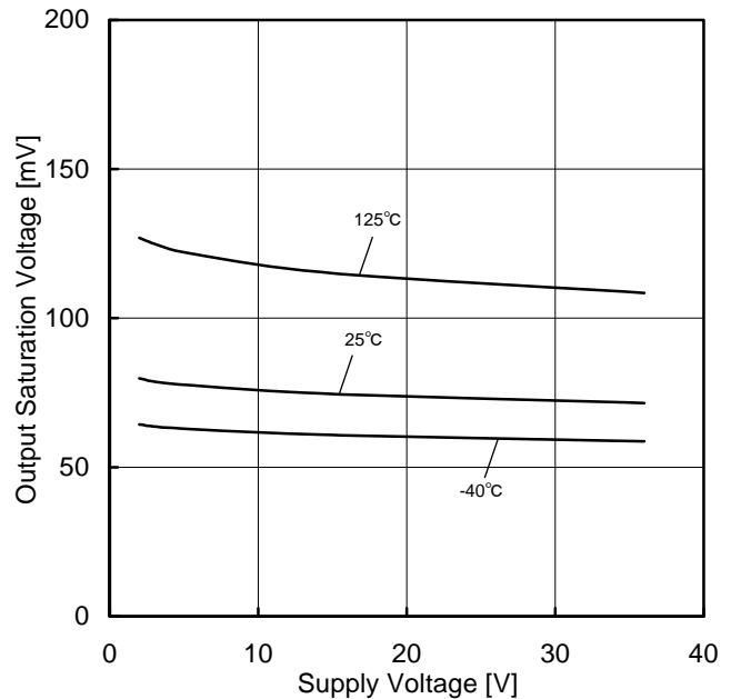
Figure 28. 出力飽和電圧—電源電圧特性 (I SINK =4mA)
