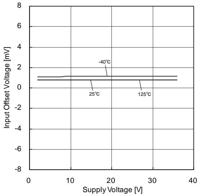
Figure 32. 入力オフセット電圧-電源電圧特性
