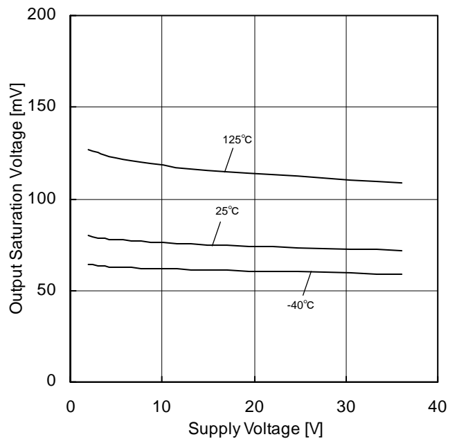
Figure 5. 出力飽和電圧－電源電圧特性 (I SINK =4mA)
