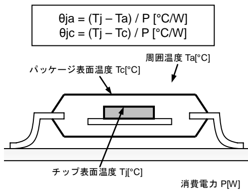
Fig.22 熱抵抗
