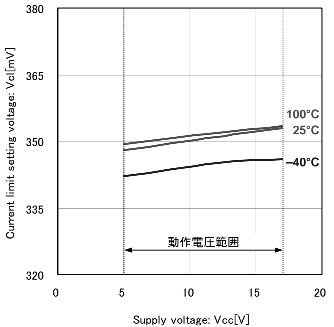
Fig.18 カレントリミット設定電圧
