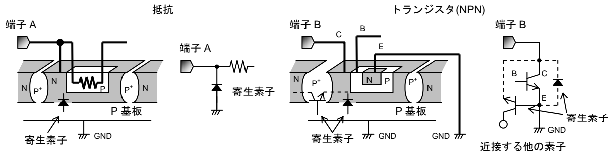
寄生素子の模式図
