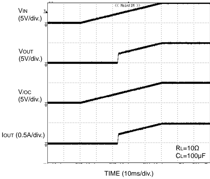
Figure 38. UVLO 特性 VIN 上昇時
