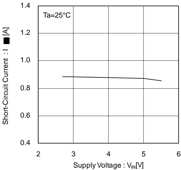
Figure 14. ショート時出力電流
