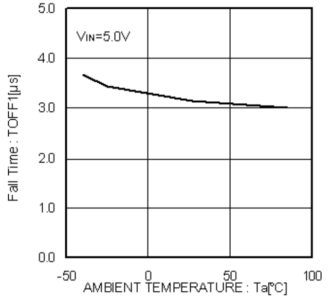
Figure 25. 出力立ち下り時間
