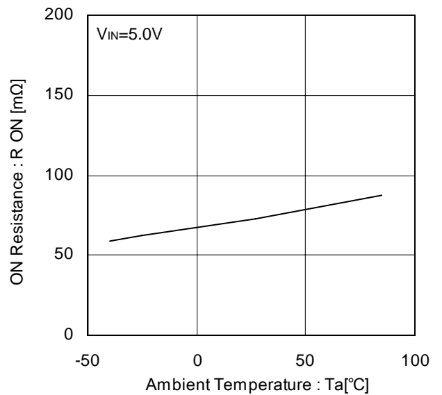
Figure 11. オン抵抗
