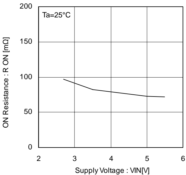
Figure 10. オン抵抗
