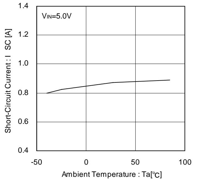
Figure 15. ショート時出力電流
