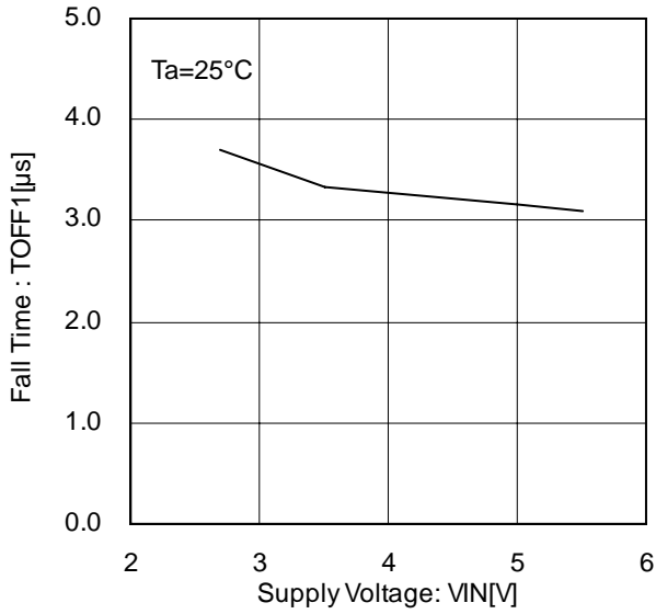
Figure 24. 出力立ち下り時間
