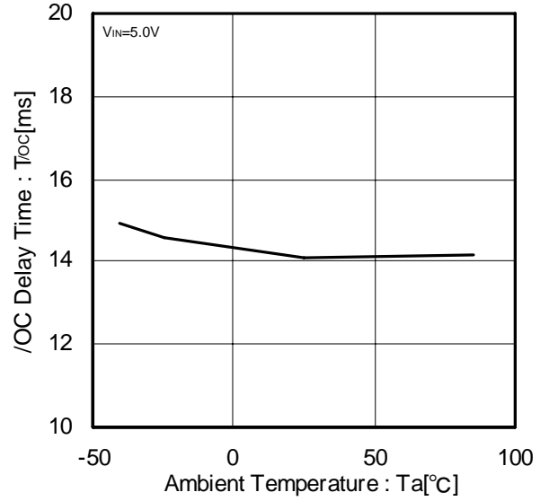
Figure 29. /OC 遅延時間
