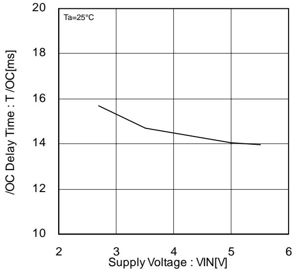
Figure 28. /OC 遅延時間
