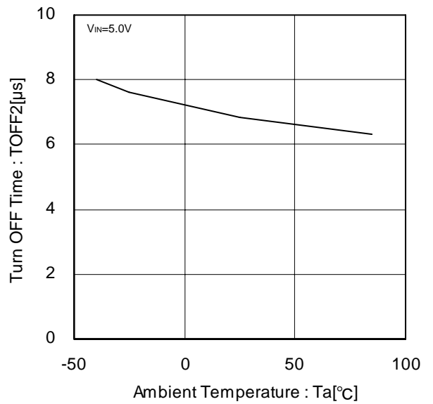
Figure 27. 出力立ち下り遅延時間
