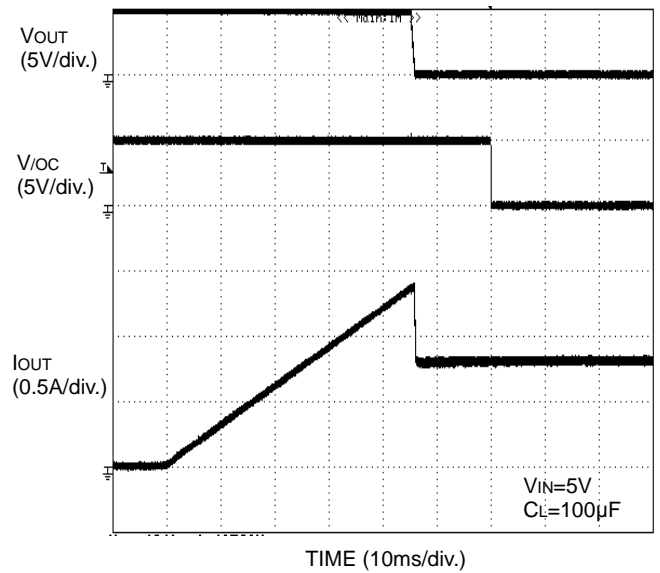
Figure 33. 過電流検出特性 ランプ出力
