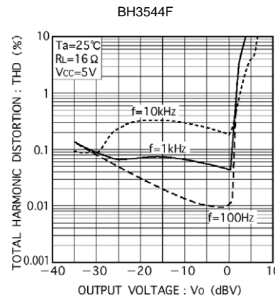
Fig. 8 全高調波歪率-出力電圧特性(4)
