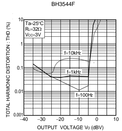
Fig. 6 全高調波歪率-出力電圧特性(2)
