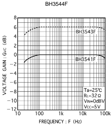
Fig. 4 電圧利得-周波数特性
