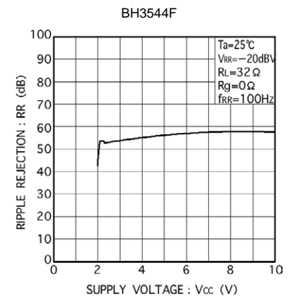
Fig. 12 リプルリジェクション-電源減圧特性
