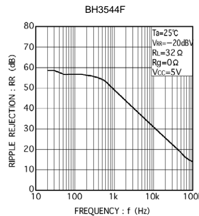
Fig. 11 リプルリジェクション-周波数特性
