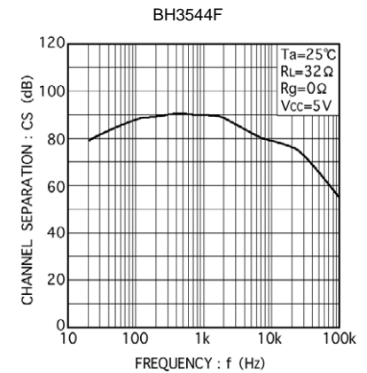
Fig. 9 チャンネルセパレーション-周波数特性
