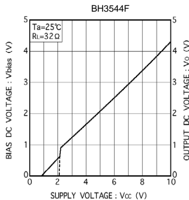
Fig. 2 端子直流電圧-電源電圧特性
