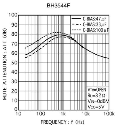
Fig. 10 ミュート減衰量-周波数特性
