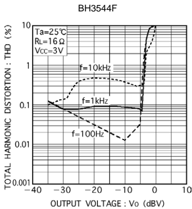
Fig. 7 全高調波歪率-出力電圧特性(3)
