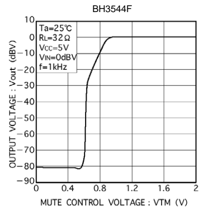
Fig. 3 出力電圧-ミュート電圧特性
