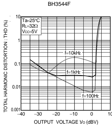
Fig. 5 全高調波歪率-出力電圧特性(1)
