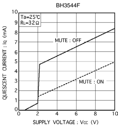
Fig. 1 無信号時回路電流-電源電圧特性
