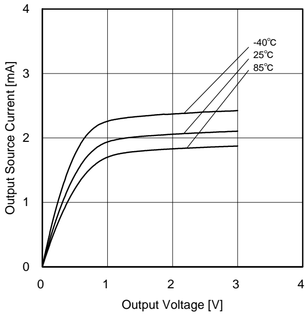
Figure 9. ローレベル出力電流 vs 出力電圧特性 ( V_{DD}=3V / V_{SS}=0V )
