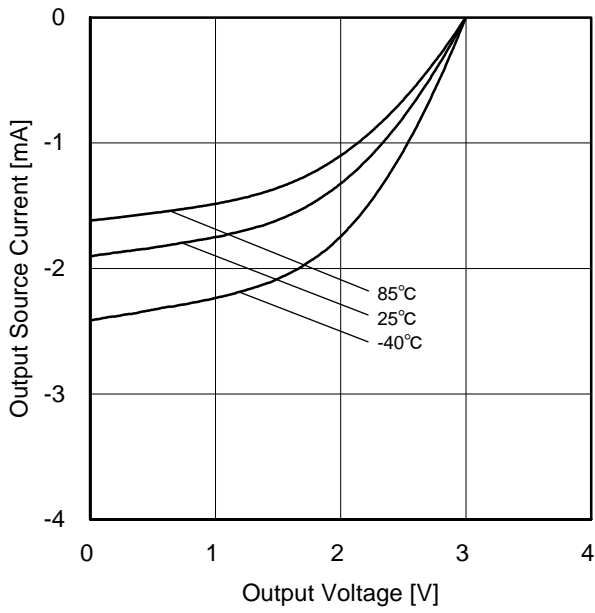
Figure 5. ハイレベル出力電流 vs 出力電圧特性 ( V_{DD}=3V / V_{SS}=0V )
