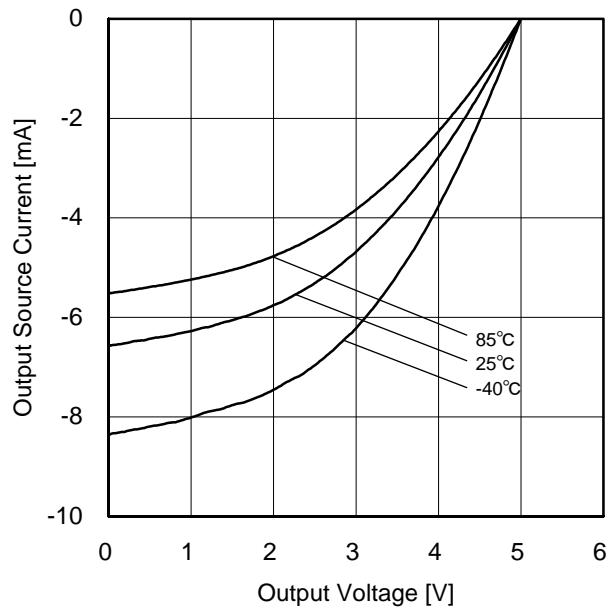
Figure 6. ハイレベル出力電流 vs 出力電圧特性 ( V_{DD}=5V / V_{SS}=0V )
