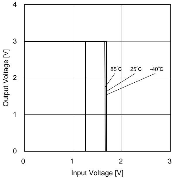
Figure 1. 出力電圧 vs 入力電圧特性 ( V_{DD}=3V / V_{SS}=0V )
