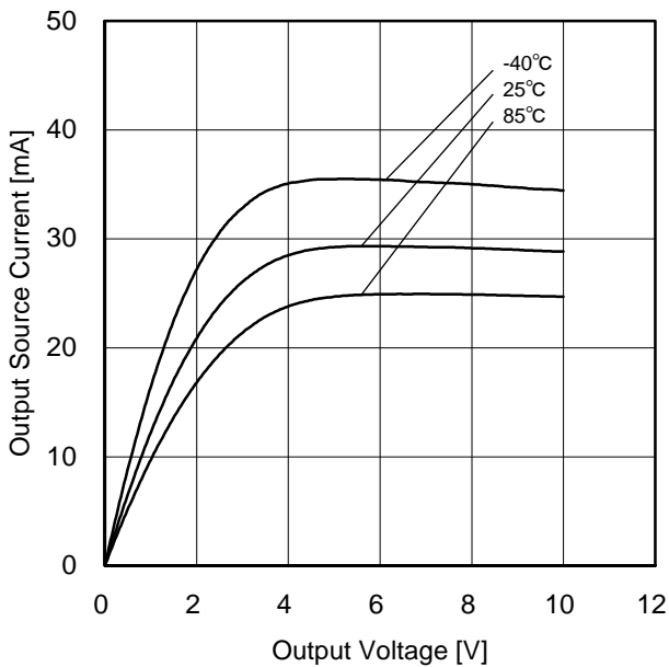
Figure 11. ローレベル出力電流 vs 出力電圧特性 ( V_{DD}=10V / V_{SS}=0V )
