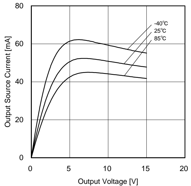
Figure 12. ローレベル出力電流 vs 出力電圧特性 ( V_{DD}=15V / V_{SS}=0V )
