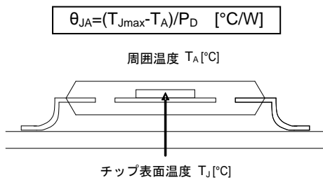
Figure 17. 熱抵抗
