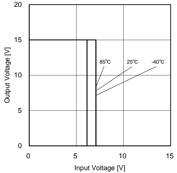
Figure 4. 出力電圧 vs 入力電圧特性 ( V_{DD}=15V / V_{SS}=0V )
