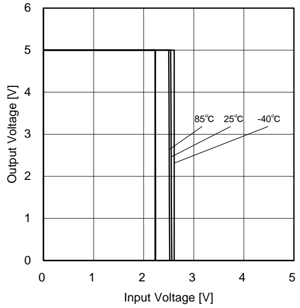
Figure 2. 出力電圧 vs 入力電圧特性 ( V_{DD}=5V / V_{SS}=0V )
