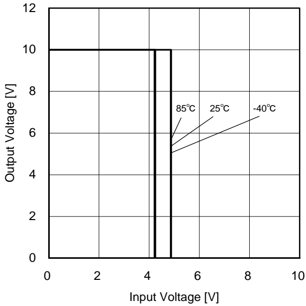
Figure 3. 出力電圧 vs 入力電圧特性 ( V_{DD}=10V / V_{SS}=0V )
