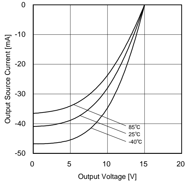
Figure 8. ハイレベル出力電流 vs 出力電圧特性 ( V_{DD}=15V / V_{SS}=0V )
