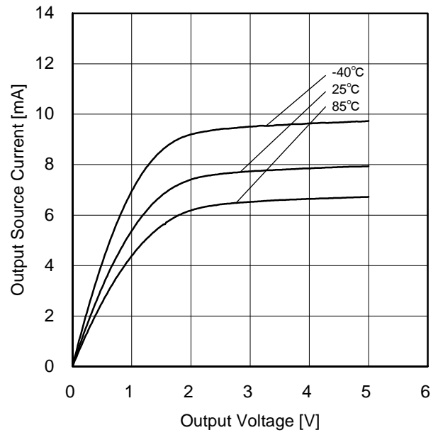
Figure 10. ローレベル出力電流 vs 出力電圧特性 ( V_{DD}=5V / V_{SS}=0V )
