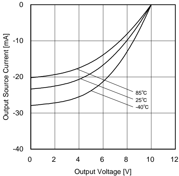
Figure 7. ハイレベル出力電流 vs 出力電圧特性 ( V_{DD}=10V / V_{SS}=0V )
